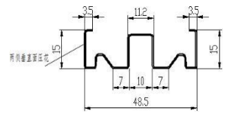
龙骨型材板型图（参考）
